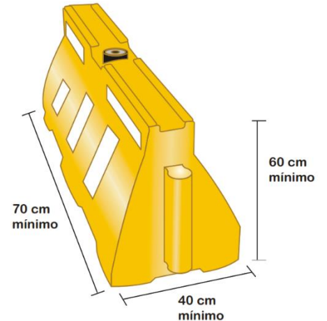
Figura 4.5 Barreras plásticas flexibles
