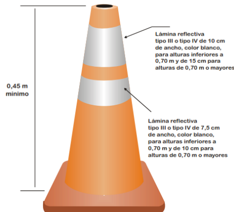
Figura 4.2 Conos
