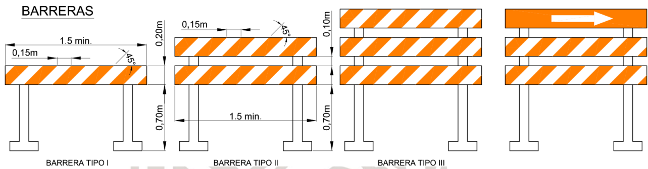
Figura 4.5 Barreras plásticas flexibles
